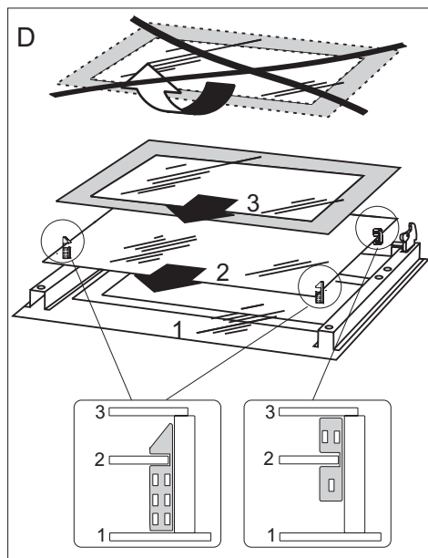
Vyberanie vnútročného skla. 3 skla.
